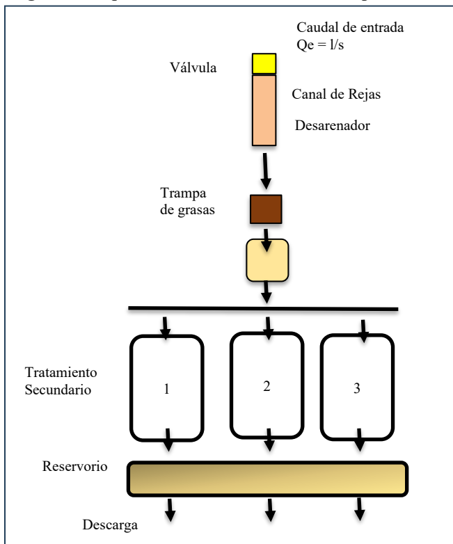
Figura 2. Esquema sistema de tratamiento tipo Wetland
